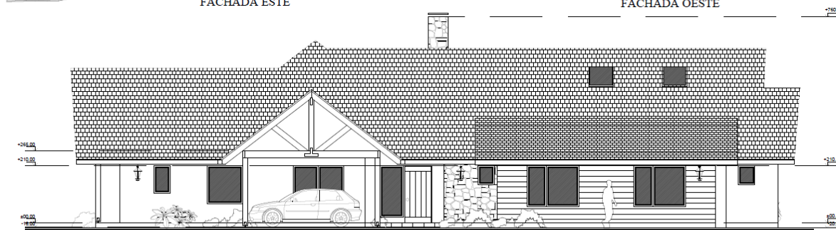
FACHADA NORTE
